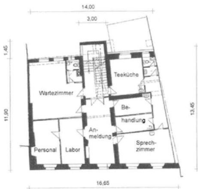
Grundriß Obergeschoß
