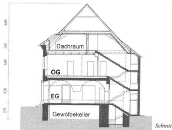
Schnitt:
