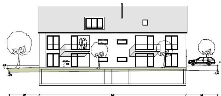
Ansicht Süd
