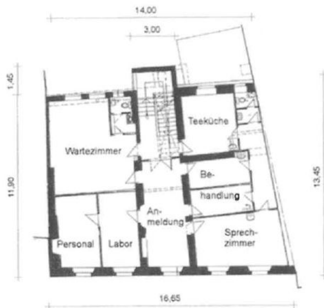
Grundriß Obergeschoß
