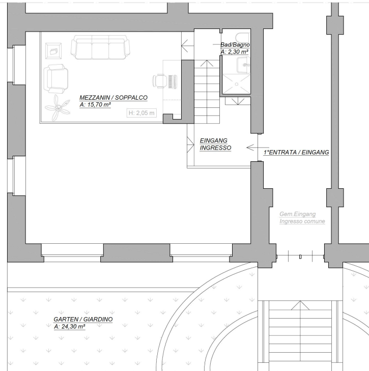
GRUNDRISS DER MEZZANINE - PLANIMETRIA SOPPALCO MEZZANIN - MEZZANINO
