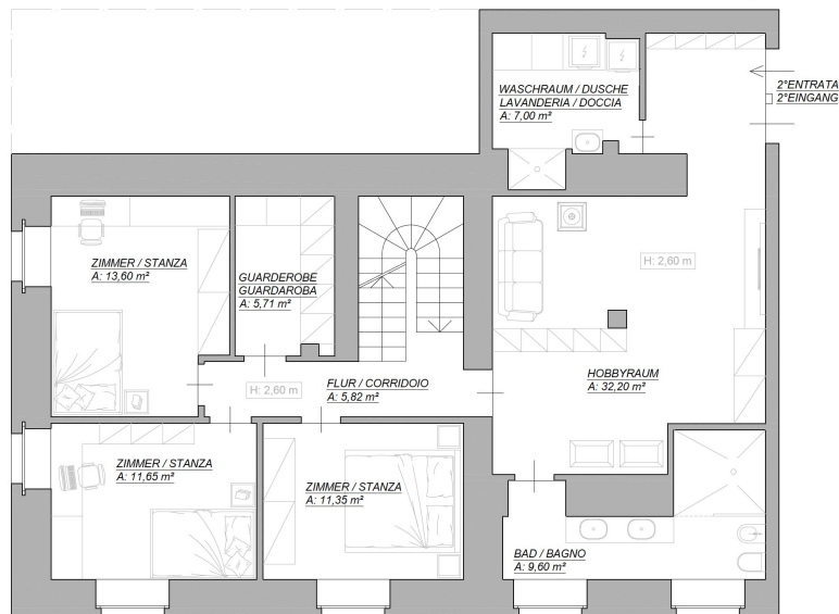
GRUNDRISS DES SCHLAFBEREICHS - PLANIMETRIA ZONA NOTTE TIEFGESCHOSS - PIANO SEMINTERRATO
