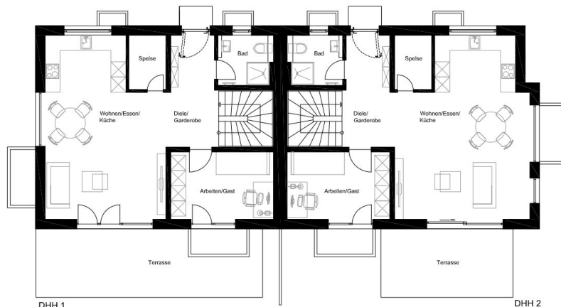
DHH 1 Grundriss EG
