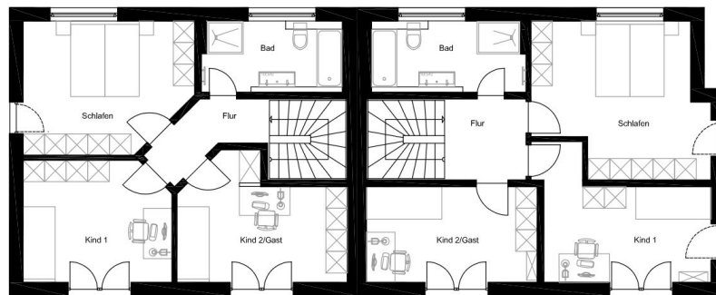
DHH 1 Grundriss OG
