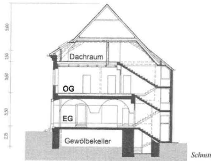
Schnitt:
