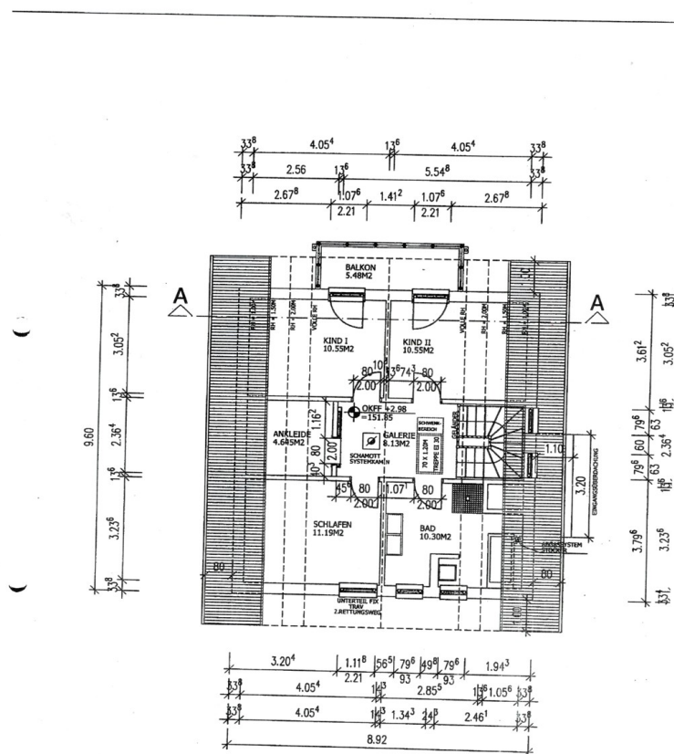
GRUNDRISS OBERGESCHOSS
