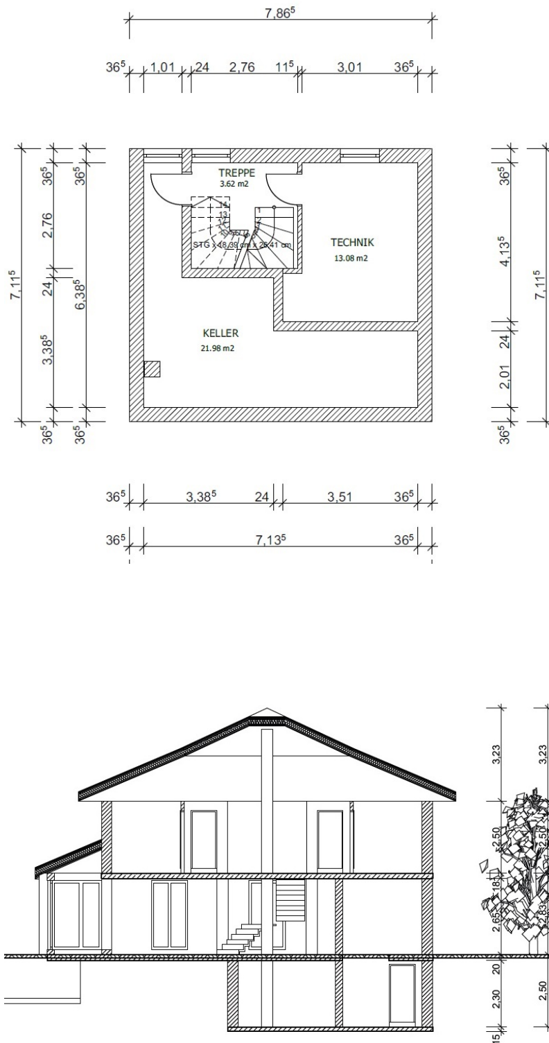
SCHNITT A - A M 1 : 100
