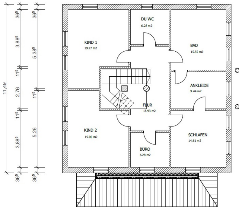
OBERGESCHOSS M 1 : 100
