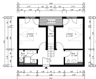
Erdbgeschoss
