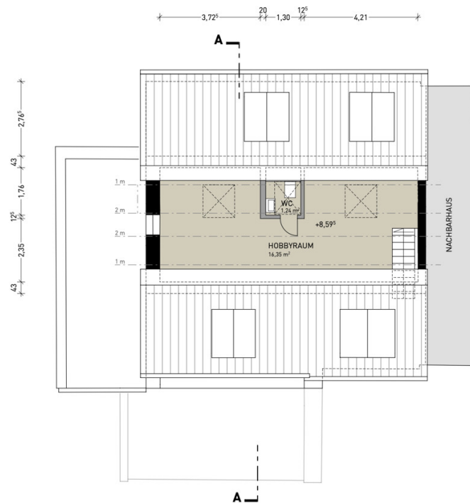
DACHBODEN
