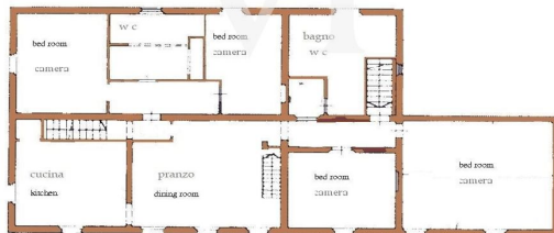
Piano primo
