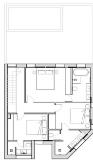
1 PRIMERA PLANTA PISO DE VIVIENDA
