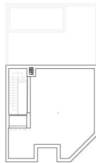
2 CUBIERTA PISO DE VIVIENDA
