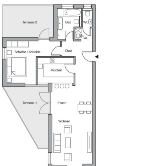
Wohnung 1 | EG Haus A
