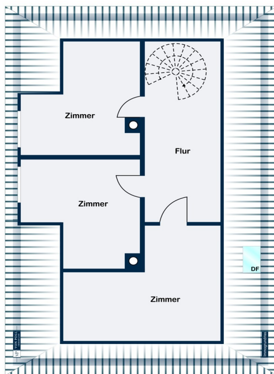
Dachgeschoss
