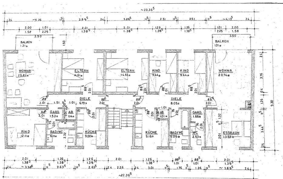
1.+2. OBERGESCHOSS M.1:100
