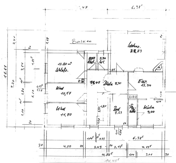
Grundriss Obergeschoss
