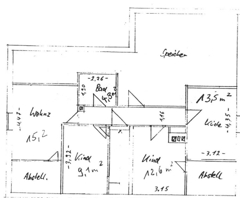
Grundriss Dachgeschoss
