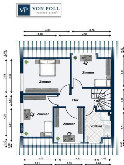
Dachgeschoss
