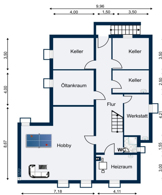
Kellergeschoss
