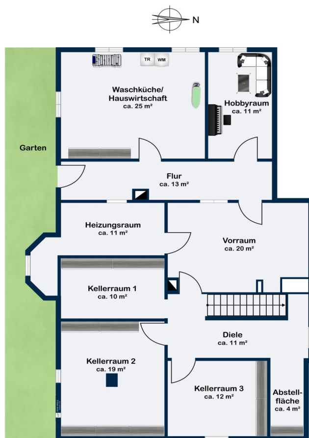
Untergeschoss
