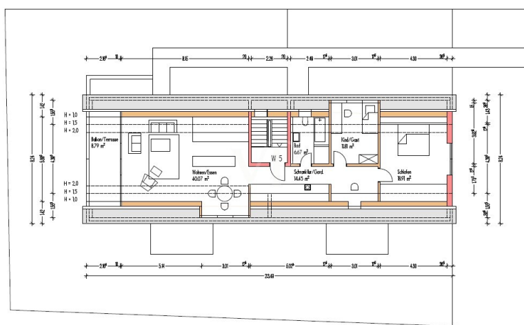
Dachgeschoss
