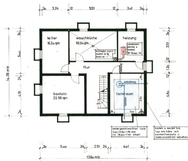
kellergeschoss
